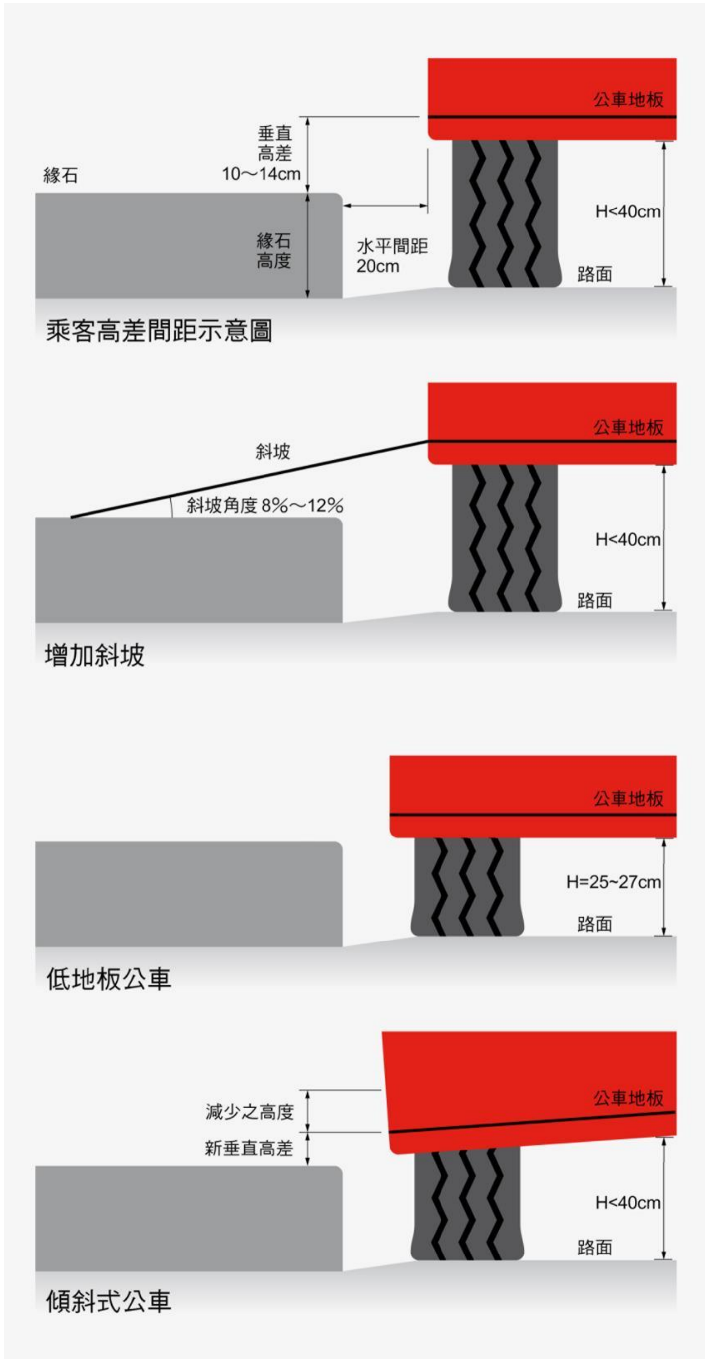
圖 9-3-6 車輛與緣石設計示意圖
