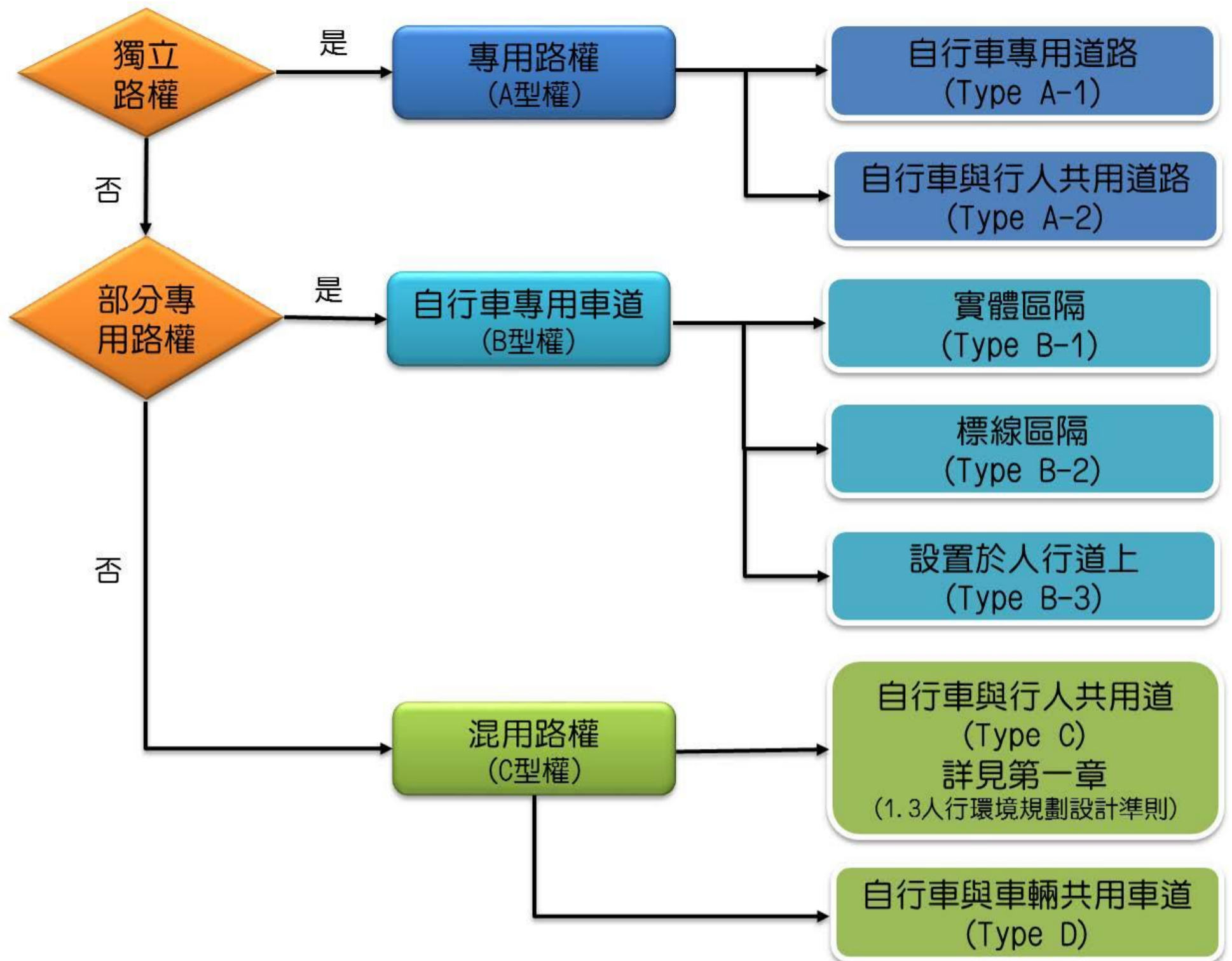
圖 7-4-1 自行車道建置類型流程圖
