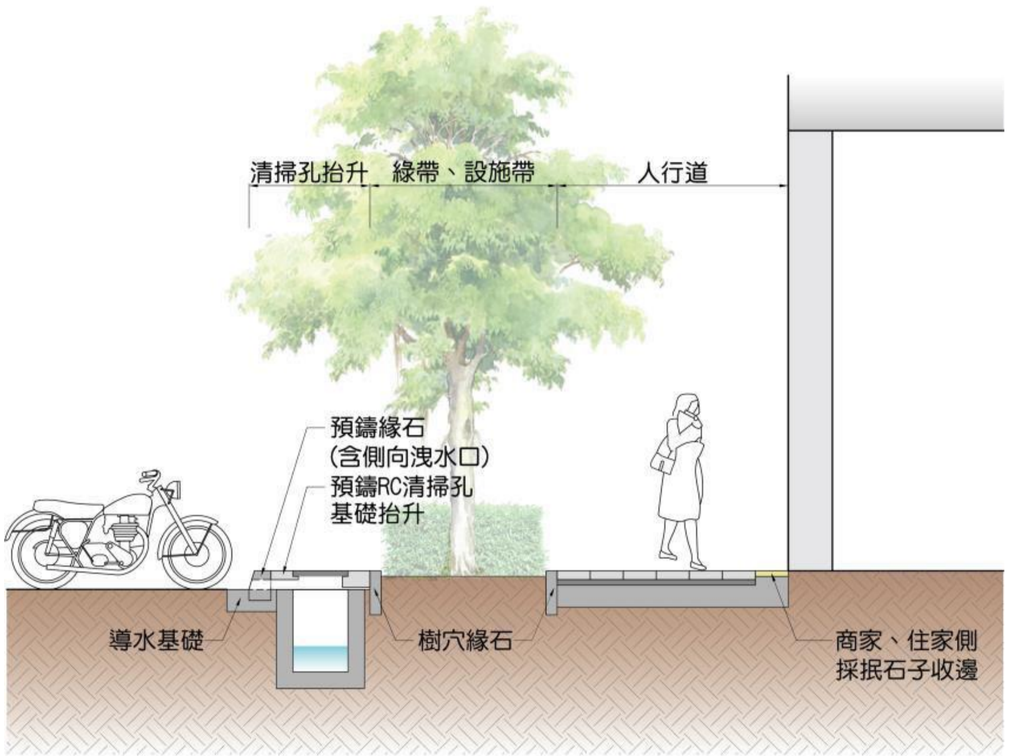
圖 4-3-32 人手孔完成面高程拉平調整案例
