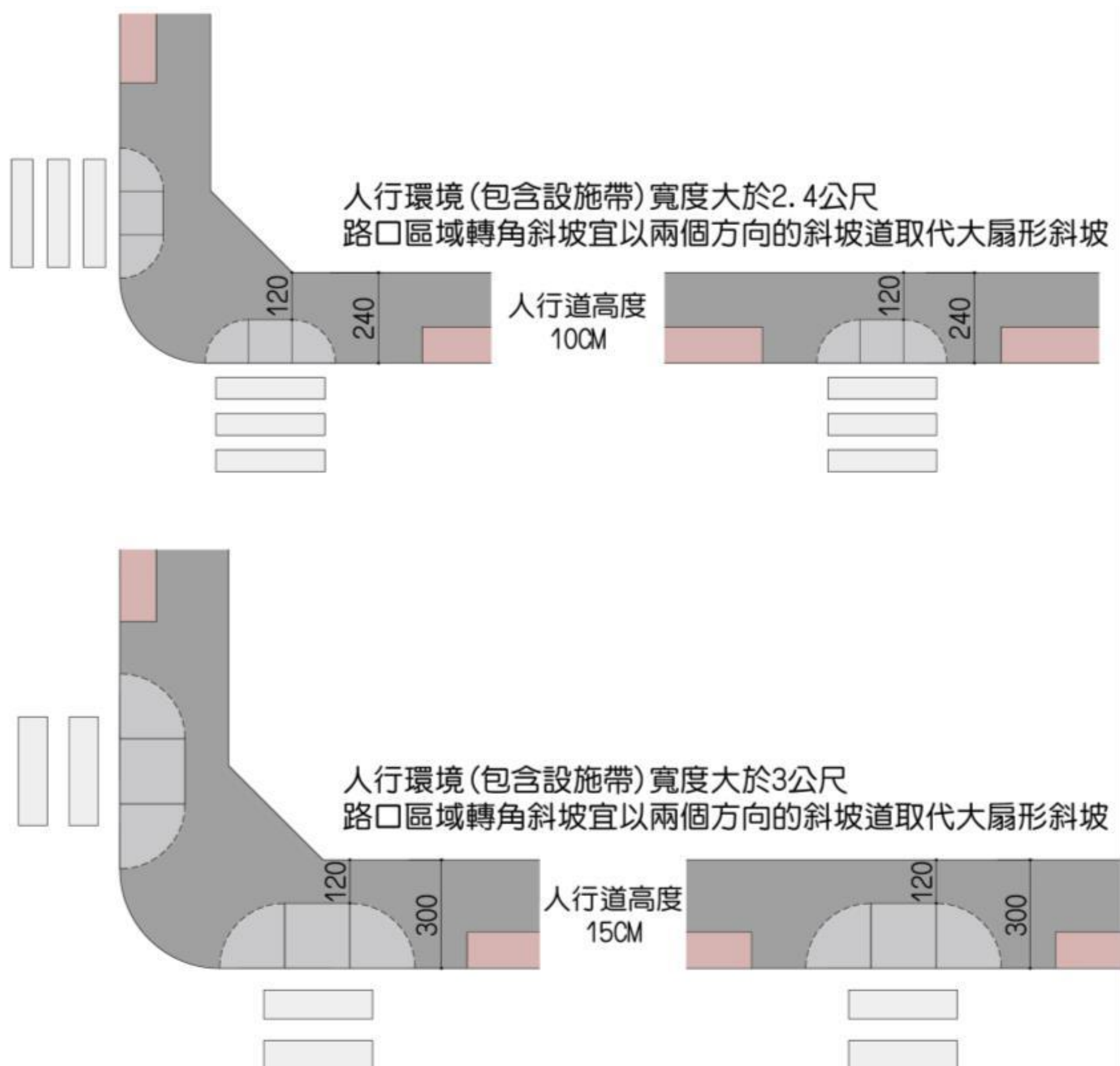
圖 4-3-21 路口轉角斜坡道設置示意圖
