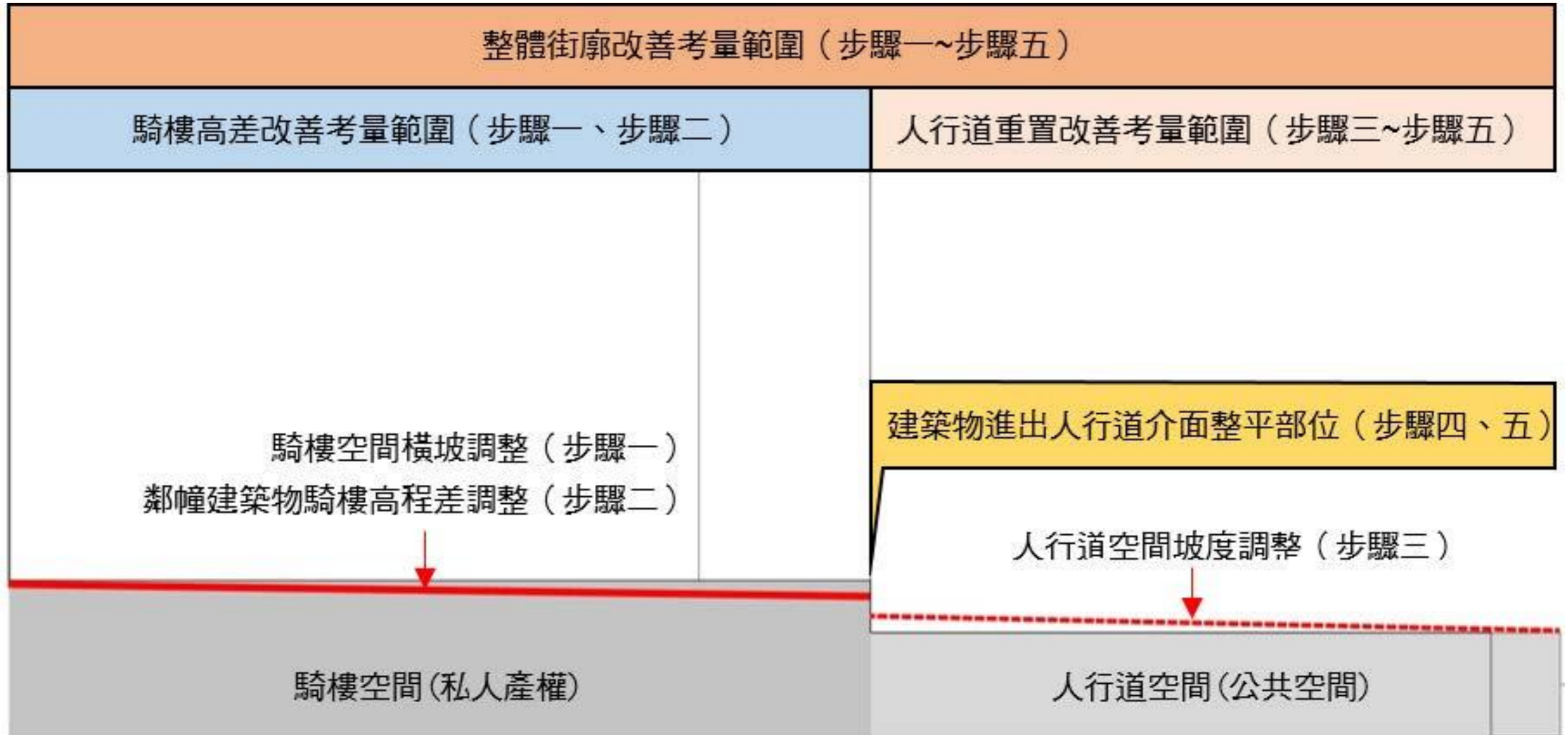
圖 4-3-3 騎樓空間整平檢討步驟示意圖
