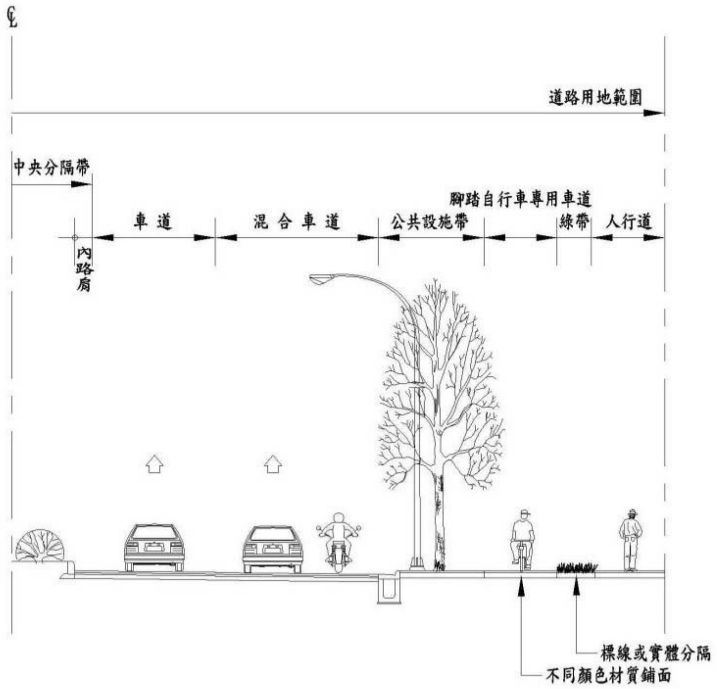
圖 5.1.1 腳踏自行車專用車道示意圖(一)
