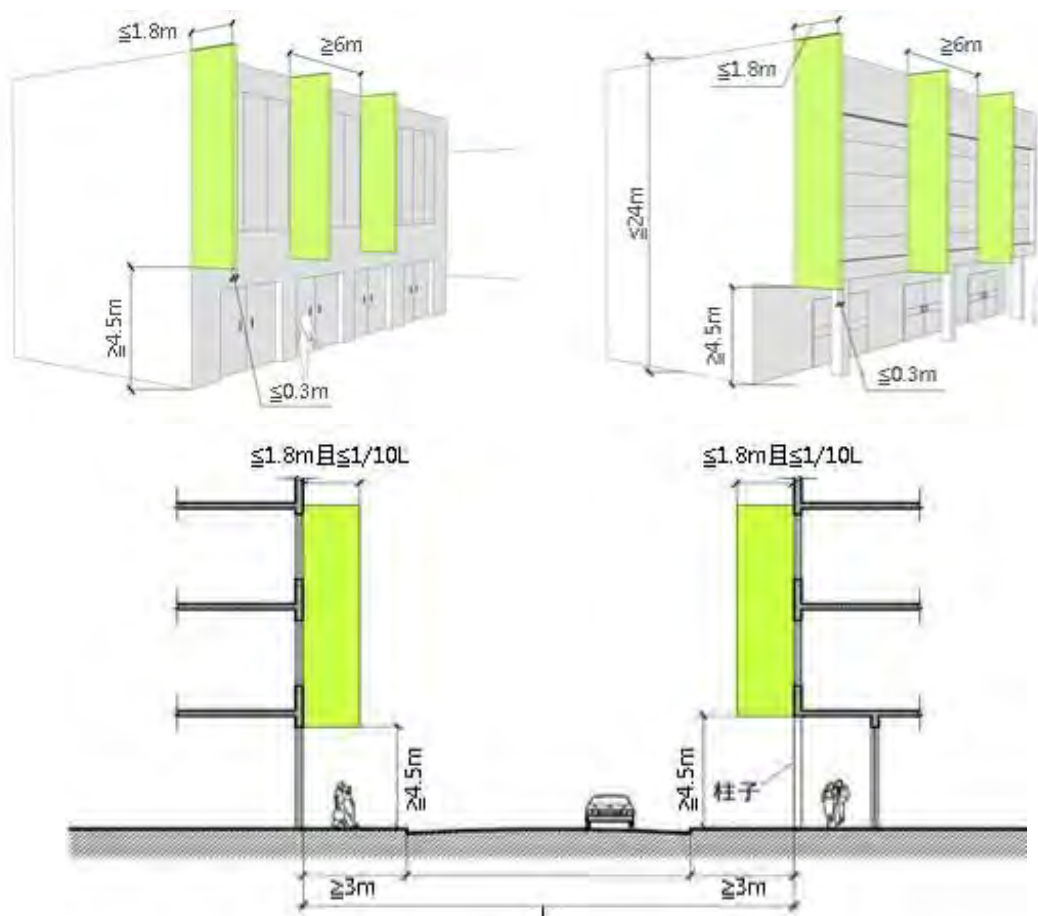
圖17 招牌牌面統一形式參考示意圖
