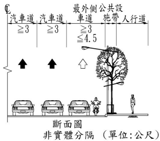
圖 2.2.2 最外側車道配置參考圖
