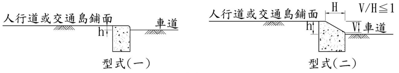
可跨式緣石
