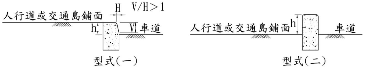
屏障式緣石
